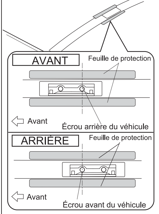
Fig-1 Emplacement d' installation des porteurs
